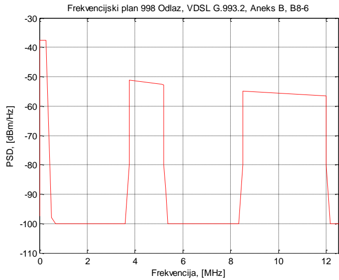
Slika 4.8.3 Maska PSD za VDSL2 frekvenijski plan 998, B8-6 odlaz (crveno)
