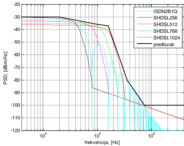
Slika 5.6.5 Frekvencijski predložak za odlazni smjer prijenosa (duge pretplatničke linije) za ADSL preko POTS (aneks A).
