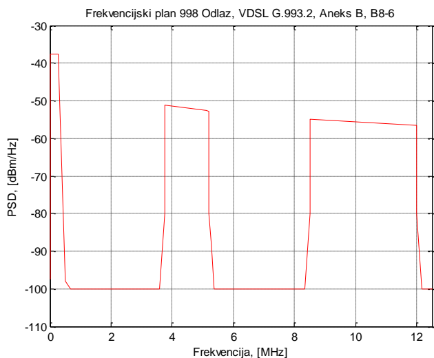
Slika 5.6.2 Frekvencijski predložak za odlazni smjer prijenosa za VDSL2, frekvencijski plan 998, B8-6
