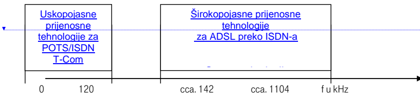
Slika 1. Frekvencijski opseg za uskopolasne i širokopolasne prijenosne tehnologije
