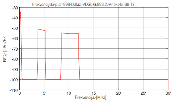
Slika 5.6.3 Frekventijski predložak za odlazni smjer prijenosa za VDSL2, frekventijski plan 998, B8-12
