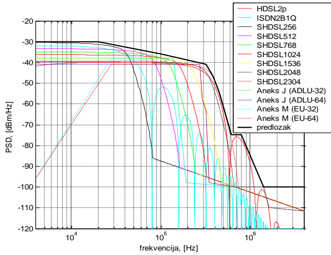
Slika 5.6.1 Frekventijski predložak za odlazni smjer prijenosa (kratke pretplatničke linije).
