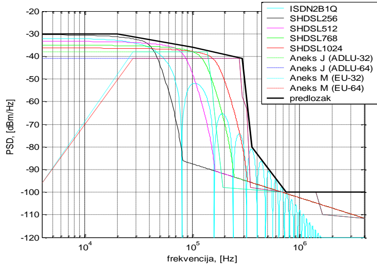
Slika 5.6.4 Frekvencijski predložak za odlazni smjer prijenosa (duge pretplatničke linije) za ADSL preko ISDN (aneks B).
