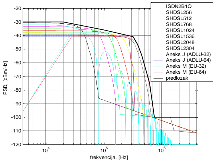
Slika 5.6.3 Frekventijski predložak za odlazni smjer prijenosa (pretplatničke linije srednje duljine).
