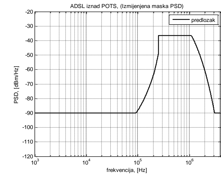
Slika 5.3.1 Frekvencijski predložak za ADSL iznad POTS (dolazni smjer).
