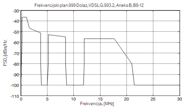
Slika 4.8.4 Maska PSD za VDSL2 frekvenijski plan 998, B8-12 dolaz (crno).
